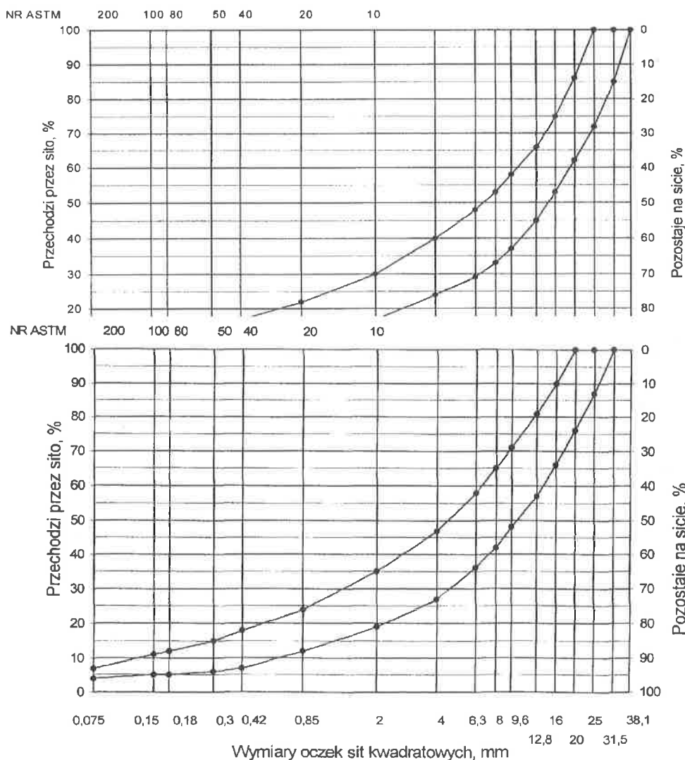
Rys. 6. Krzywe graniczne uziarnienia mieszanki mineralnej BA od 0 do 31,5 mm podbudowy nawierzchni drogi o obciążeniu ruchem od KR 3 do KR 6
